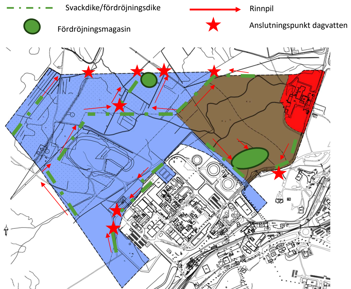
Figur 15: Framtida dagvattenhantering.
